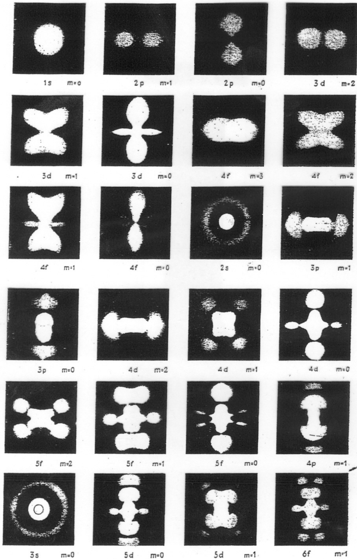
Abb. 109. Wellenmechanische „Bilder“ des H-Atomelektrons in seinen verschiedenen Anregungszuständen (Elektronenwolken) nach WHITE. Die Helligkeit gibt die Größe der Aufenthaltswahrscheinlichkeit des Elektrons an jeder Stelle an.
