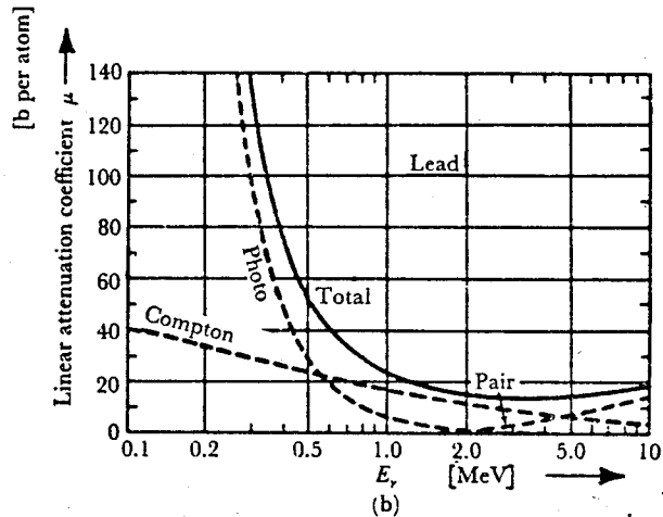
Fig. 3-21: Die Energieabhängigkeit der linearen Absorptionskoeffizienten
