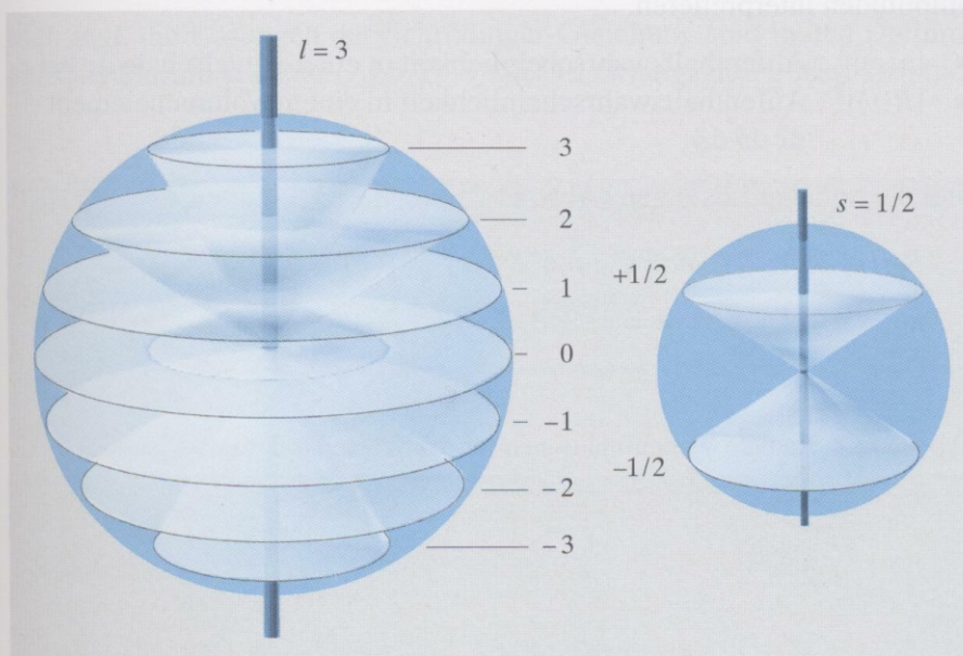
Abb. 13.5. Richtungsquantelung des Drehimpulses im Vektormodell
