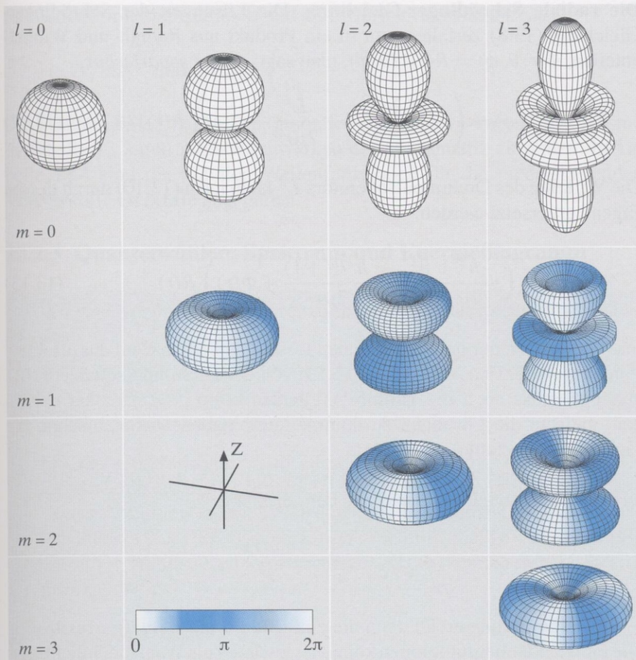
Abb. 13.4. Kugelflächenfunktionen. Die Phasenabhängigkeit ist mit der weiß-blauen Farbskala veranschaulicht
