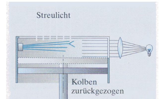
Abb. 13.36. Wilson-Kammer, schematisch
